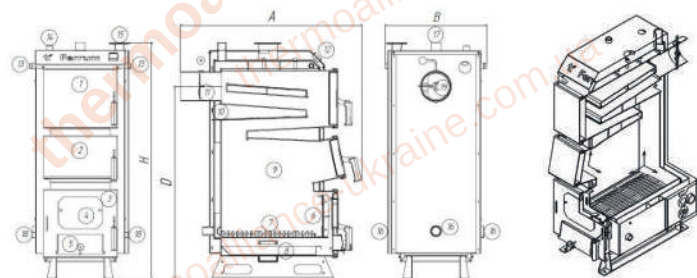
Рис.2 Ferrum FSF20, FSF26 та його конструкція:
