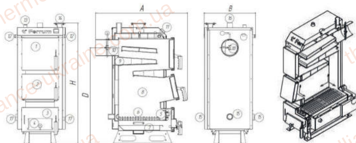
Рис.1 Ferrum FSF12, FSF16 та його конструкція:
