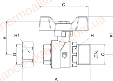
Таблиця 18. Кран кульовий з накидною гайкою, прямий, всередину-назовні ручка - метелик SF260W SD FORTE
