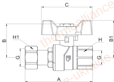
Таблиця 17. Кран кульовий з накидною гайкою, прямий, всередину-всередину ручка - метелик SF260W SD FORTE
