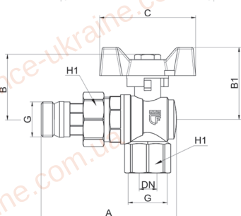
Таблиця 14. Кран кульовий зі згоном та EPDM кільцем від протікання, угловий ручка - метелик SF223W SD FORTE
