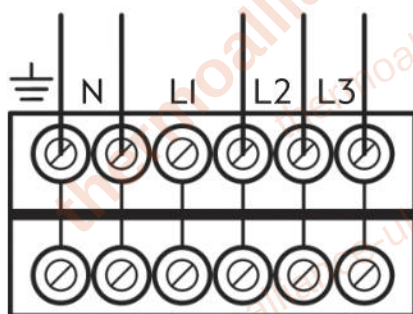
Під'єднання 380В
