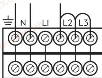
Під'єднання 220В
