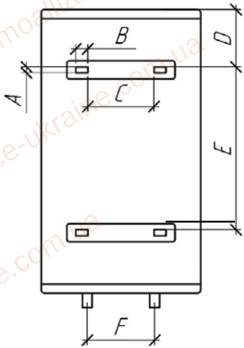
Схема монтажу та розміри
