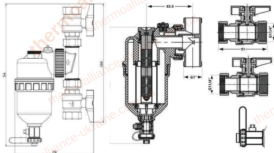
Креслення TAF400G32
