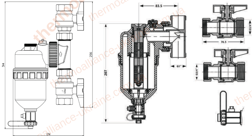
Креслення TAF400G20
