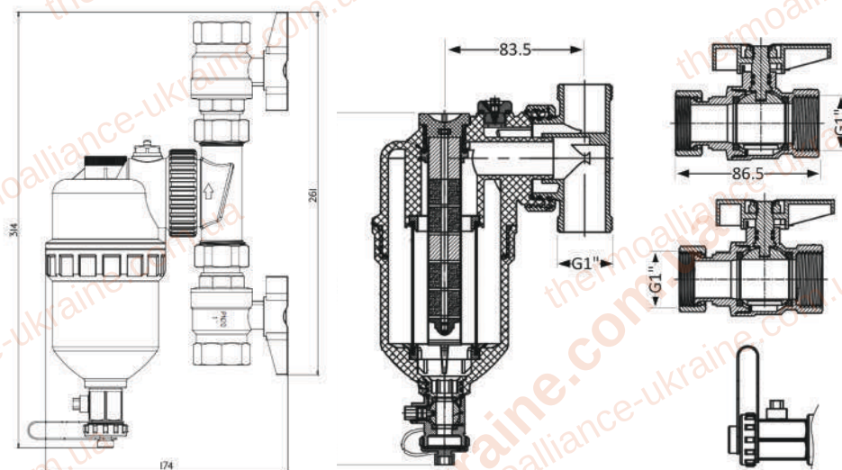
Креслення TAF400G25
