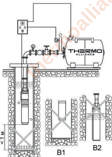
Некоректний монтаж (В)
