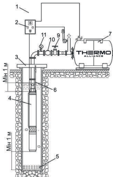
Коректний монтаж (А)
