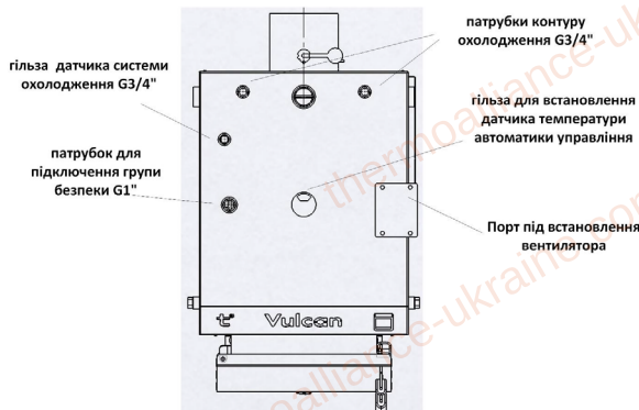
Рис.4 Патрубки для підключення та приблизна схема реалізації опції теплового розвантаження
