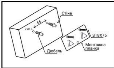
Схема монтажу
